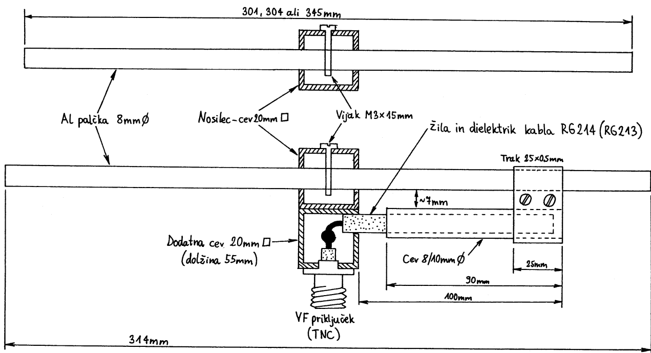
Slika 2 - Pritrditev elementov na nosilec in izvedba "gama" prilagoditve.
