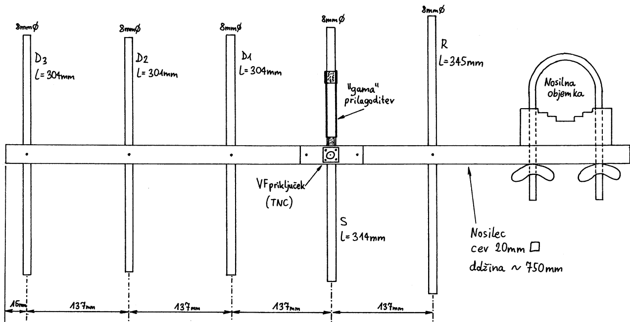
Slika 1 - 5-elementna Yagi antena za 435MHz (NBS 0.8\lambda Yagi).
